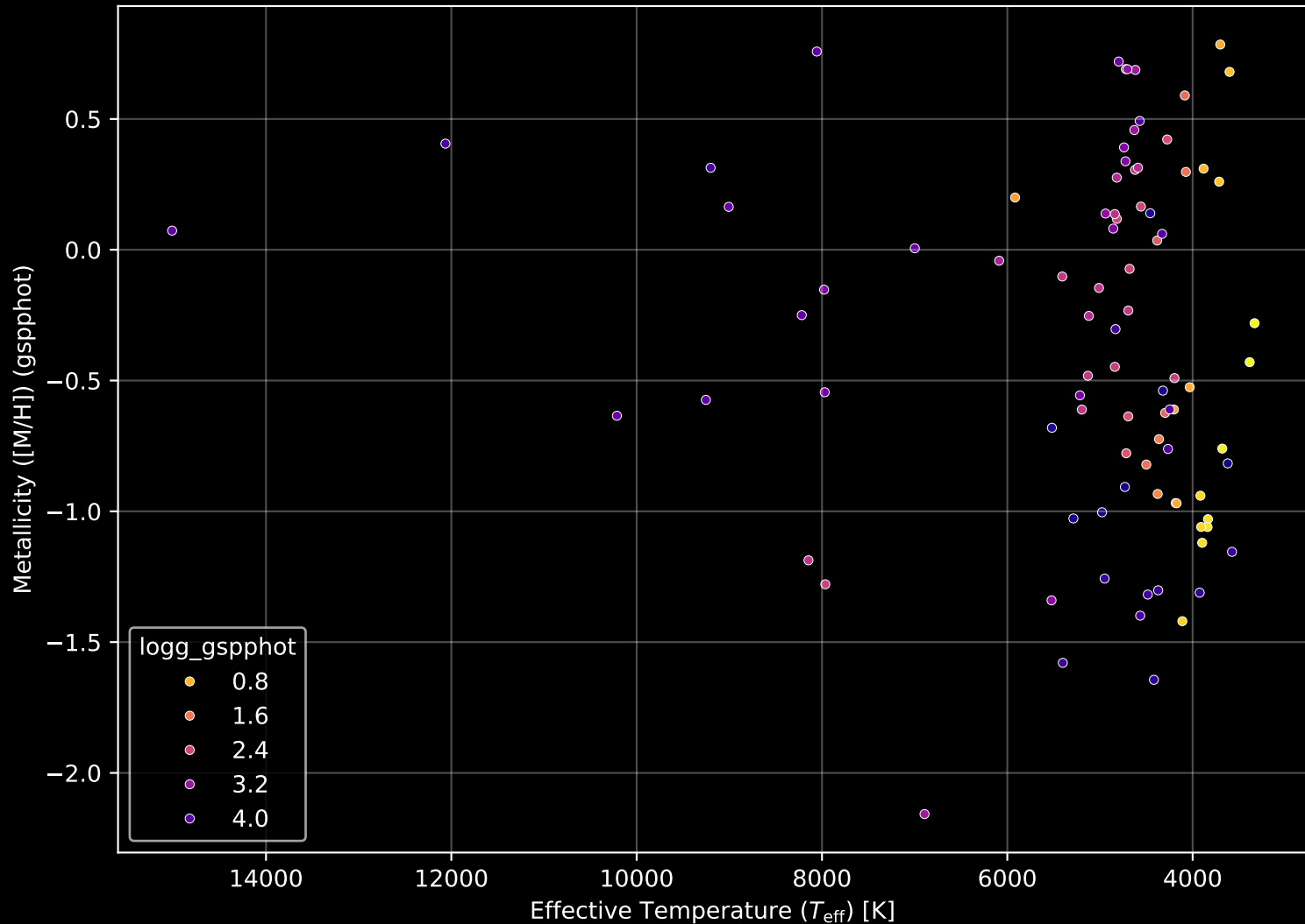
APOGEE DR17 Field: [350+00] Stellar Population Parameters (n= 89)
